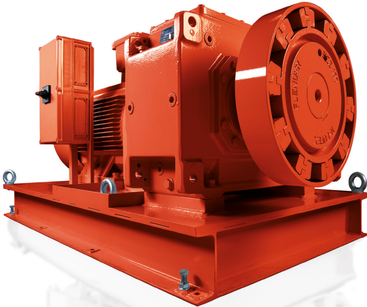
Antriebseinheit
