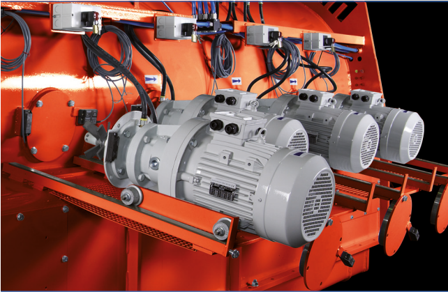
Wirblerschnellwechselsystem optional
